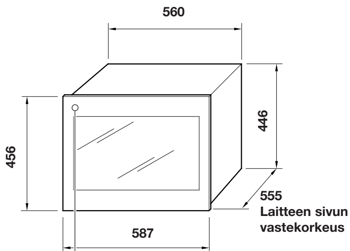
Kaapin mitat
