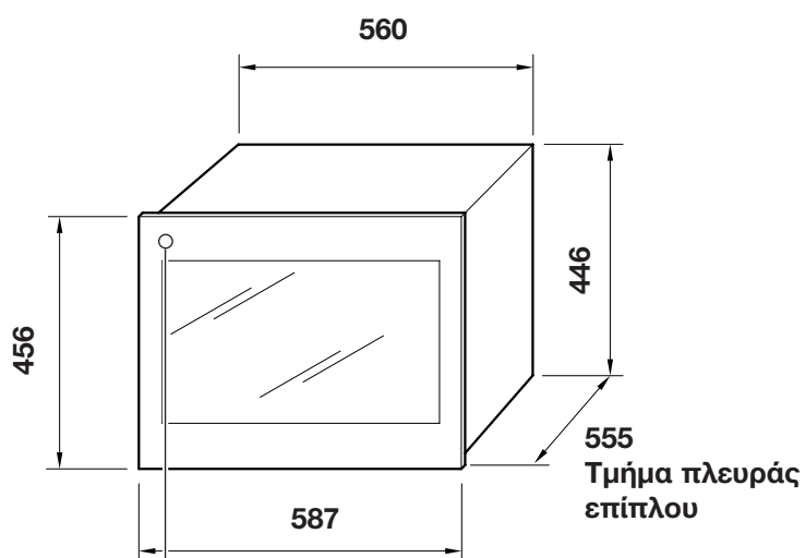
Διαστάσεις του συντηρητή
