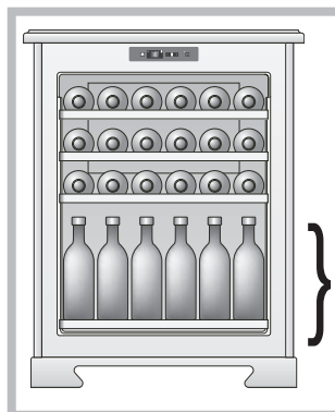
SERWOWANIE 42 butelki (50% położone i 50% postawione) z użyciem 3 półek
