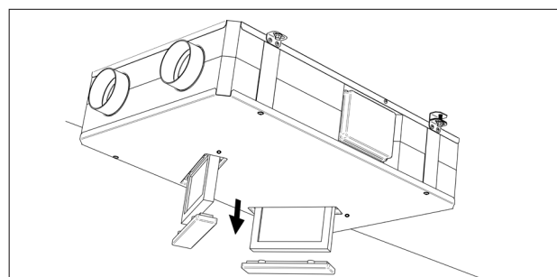
Fig. 8.f Rimuovere i tappi utilizzando la staffa in dotazione.
