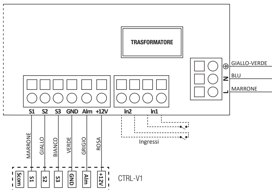
Fig. 5.k Collegamenti elettrici sulla scheda madre fissata all'interno della scatola collegamenti elettrici
