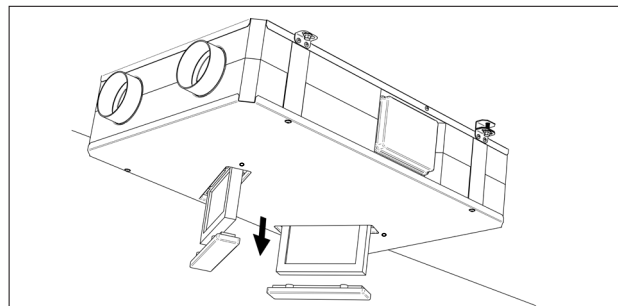
Fig. 8.c Rimuovere i tappi utilizzando la staffa in dotazione.
